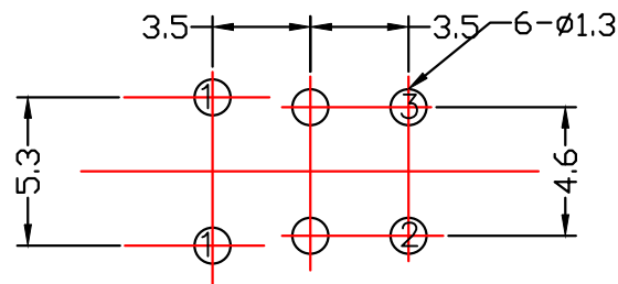
P.C.B. TERMINAL POSITION
