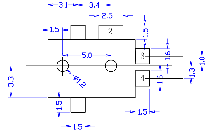
P.C.B LAND
