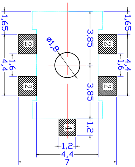
P.C.B LAND
