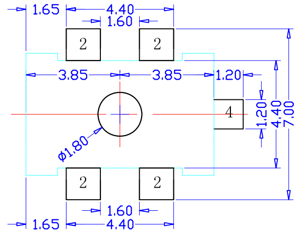
P.C.B LAND
